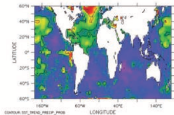
HadISST & GPCP data
